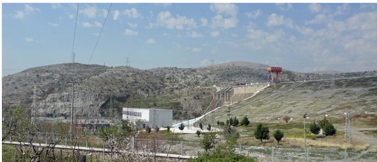
Figura 9.2: Diga e Vau të Dejës që tregon stacionin e turbinës dhe nënstacionin elektrik
