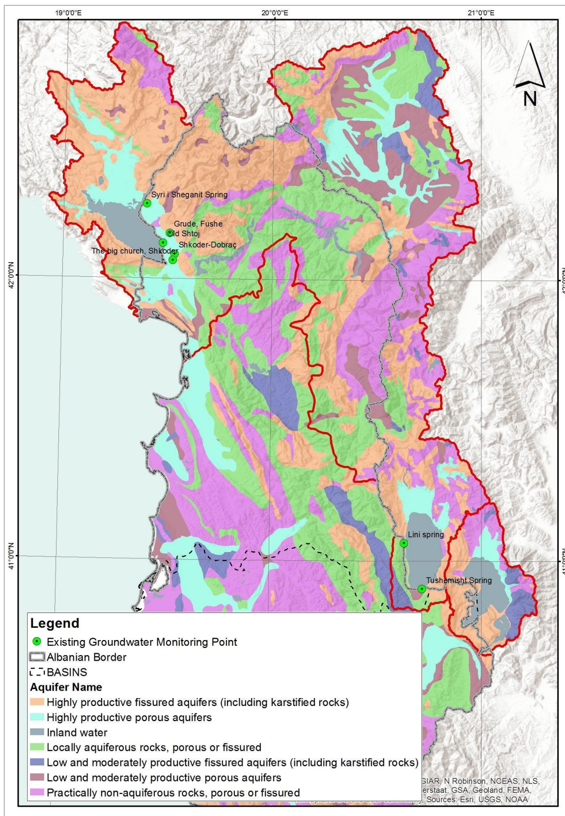
Figura 3.8: Akuiferët kryesorë të Basenit Ujor Drin-Bunë
