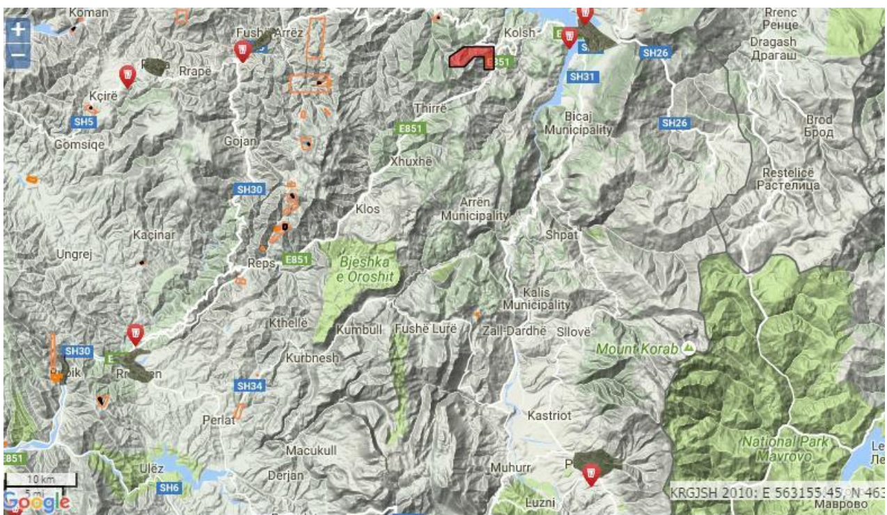
Figura 4.3: Treguesit në hartë tregojnë depozitat; zonat e kuqe dhe portokalli i referohen zonave të rrezikshme minerare
